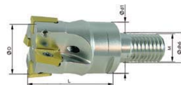
Suministro sin plaquitas de corte.
