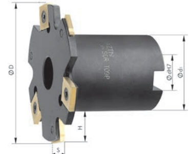
Suministro sin plaquitas de corte.
